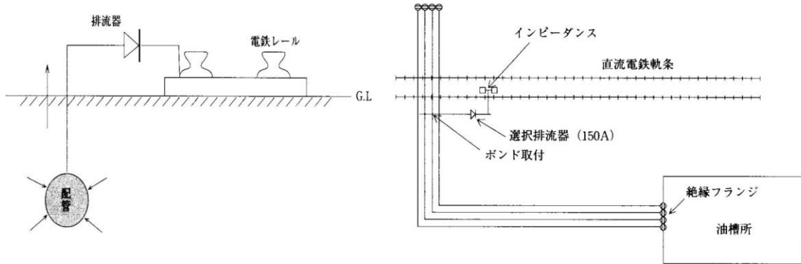
図 6 排流法
