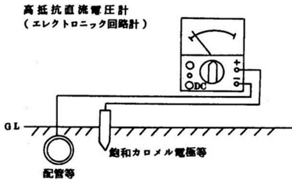
図 2 対地電位測定
