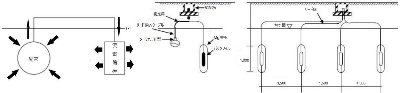
図 4 流電陽極方式
