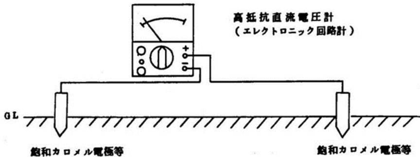
図 3 地表面電位勾配測定
